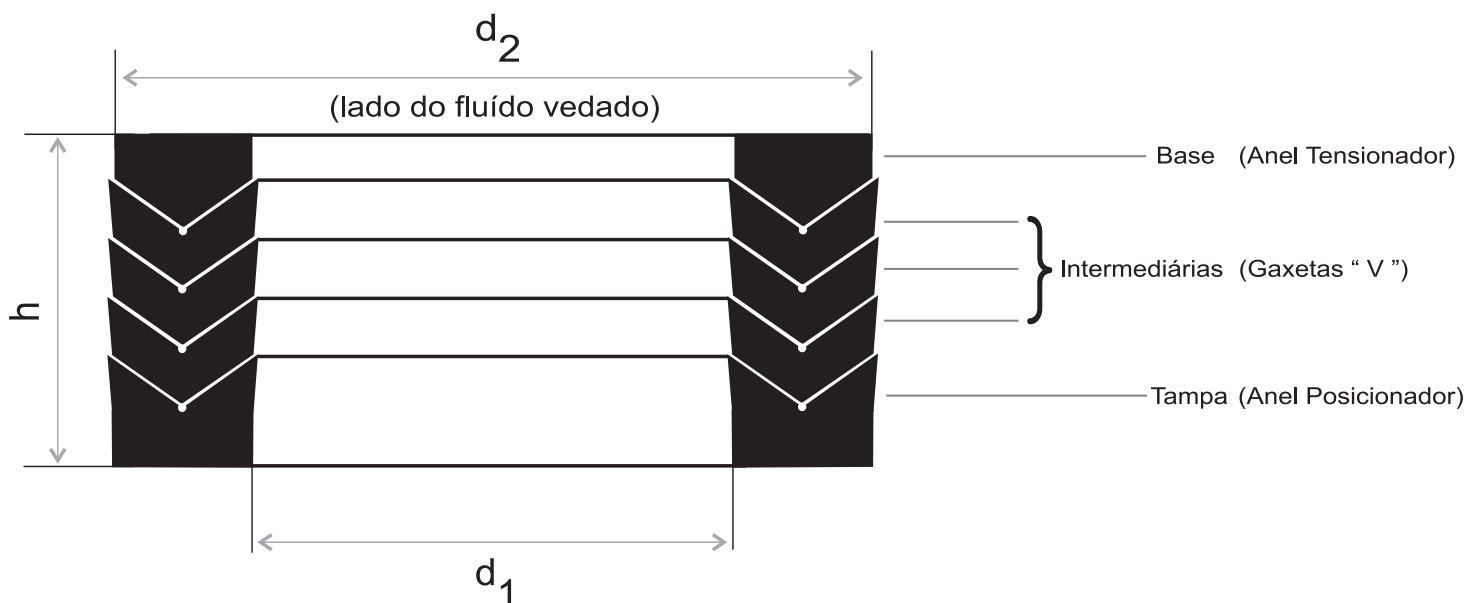
Seção de jogo de Gaxetas tipo “Chevron”
